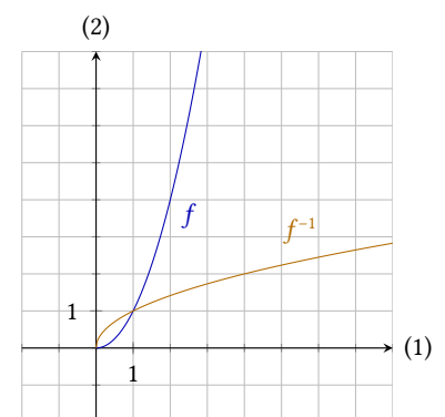
Figur 1.10: Funktionen f(x) = x^2 ( x > 0 ) og dens inverse f^{-1}(x) = \sqrt{x} .
