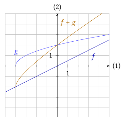
Figur 1.4: Graferne for f , g og f + g .
