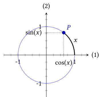
Figur 7.2: Definitionen på \cos(x) og \sin(x) .
