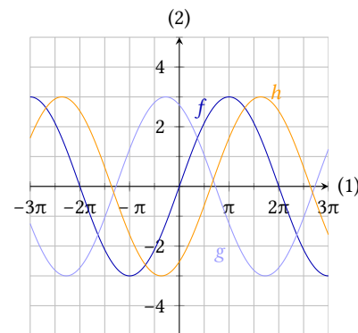
Figur 7.9: Graferne for f(x) = 3 \sin\left(\frac{1}{2}x\right) , g(x) = 3 \sin\left(\frac{1}{2}x + 2\right) og h(x) = 3 \sin\left(\frac{1}{2}x - 1\right) .
