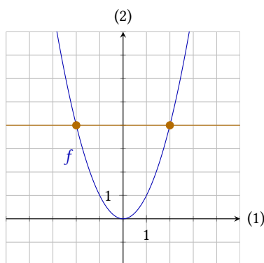
Figur 1.9: Funktionen f(x) = x^2 er ikke injektiv.
