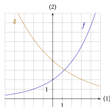
Figur 3.1: Graferne for de to eksponentielle funktioner f(x) = 2 \cdot 1,4^x og g(x) = 4 \cdot 0,8^x .
