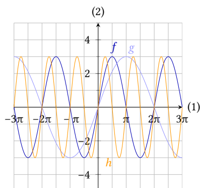
Figur 7.8: Graferne for f(x) = 3 \sin(x) , g(x) = 3 \sin\left(\frac{1}{2}x\right) og h(x) = 3 \sin(2x) .
