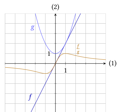
Figur 1.5: Graferne for f , g og \frac{f}{g} .
