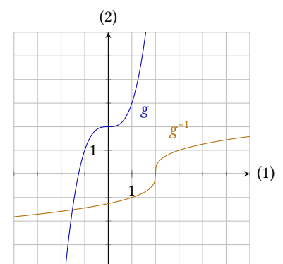
Figur 1.11: Funktionen g(x) = x^3 + 2 og dens inverse g^{-1}(x) = \sqrt[3]{x - 2} .
