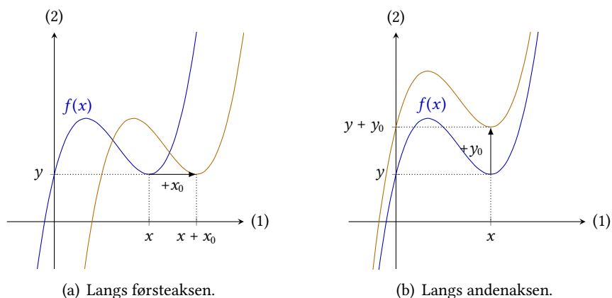
Figur 1.7: En graf kan parallelforskydes både langs første- og andenaksen.
