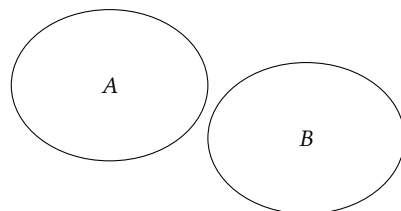
Figur A.9: A og B er disjunkte.
