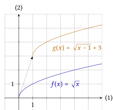
Figur 1.8: Grafen for f(x) = \sqrt{x} forskudt med (1, 3) .
